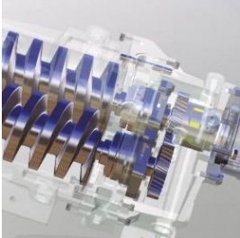
スクリー式ドライ真空ポンプ
